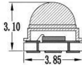
截面图
