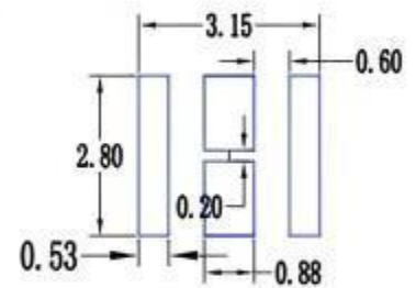
推荐钢网
