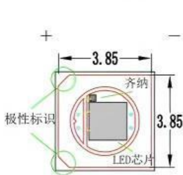
俯视图
