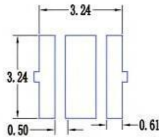
推荐焊盘
