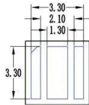
底部焊盘
